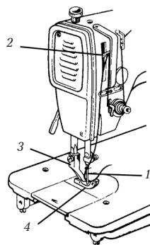
Робочі елементи швейної машини
